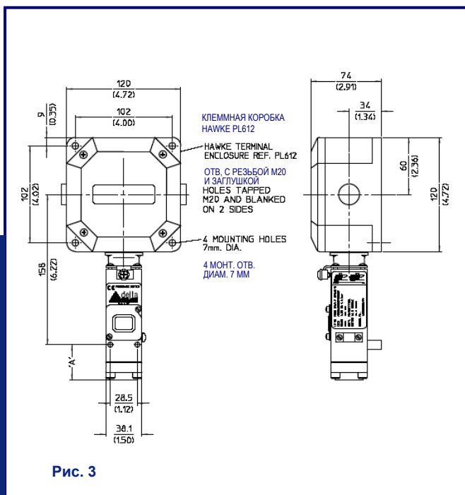
КОРПУСА КОД Н, R ТАБЛИЦА 1 С КЛЕММНЫМИ КОРОБКАМИ КОД J ТАБЛИЦА 3
