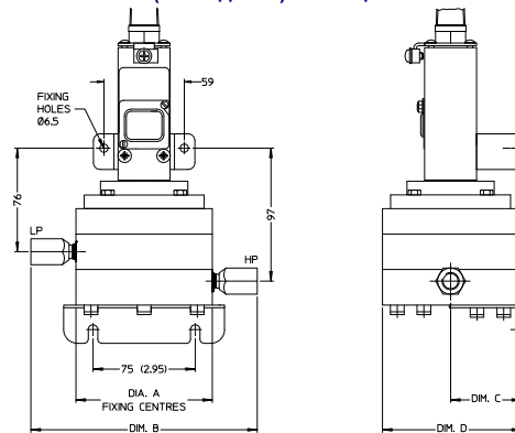
МОДЕЛЬ GR6 ДИАПАЗОНЫ от BD до EA / от 0D до EA (от 0Y до EH) Таблица 5
